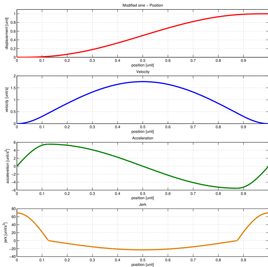
Obrázek 1.3: Modified sine
